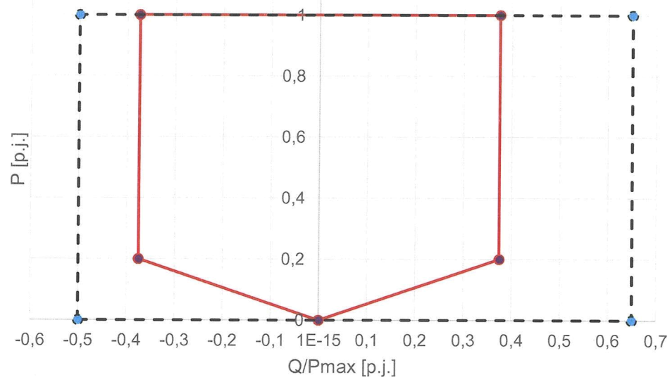
Obr. 13 Diagram dodávky jalového výkonu při nižší než maximální dodávce činného výkonu pro nesynchronní výrobní moduly kategorie D
