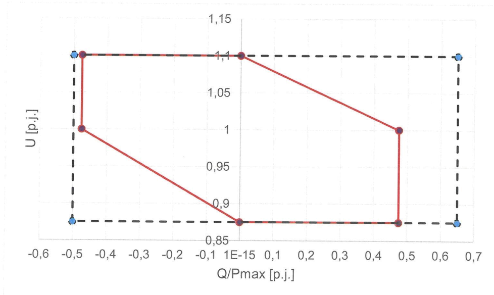
Obř. 1 Diagram dodávky jalového výkonu při maximální dodávce činného výkonu pro synchronní výrobní moduly kategorie D
