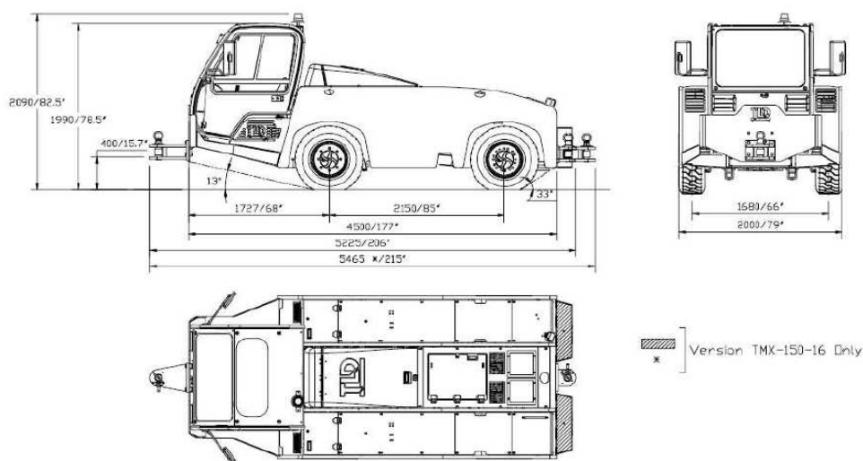
Obr. 1) Schematický náčrtek
